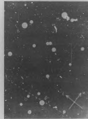
Estrellas que forman parte de la constelación de los gemelos.
